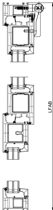
1 VANTAIL + FIXE
