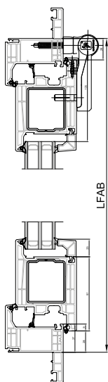
1 VANTAIL
